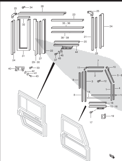
FIG. 116 DOOR GLASS RUN
