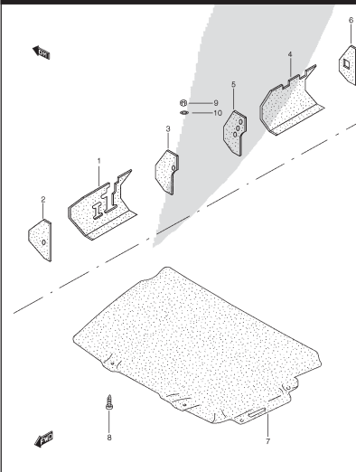
FIG. 117 SILENCER
