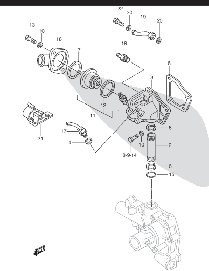
FIG. 29 THERMOSTAT
