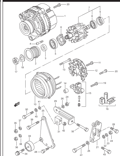
FIG. 54 GENERATOR
