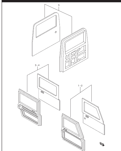
FIG. 86 DOOR PANEL
