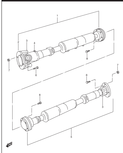
FIG. 46 PROPELLER SHAFT
